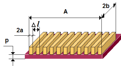
Fig. 5. Linear antenna array
